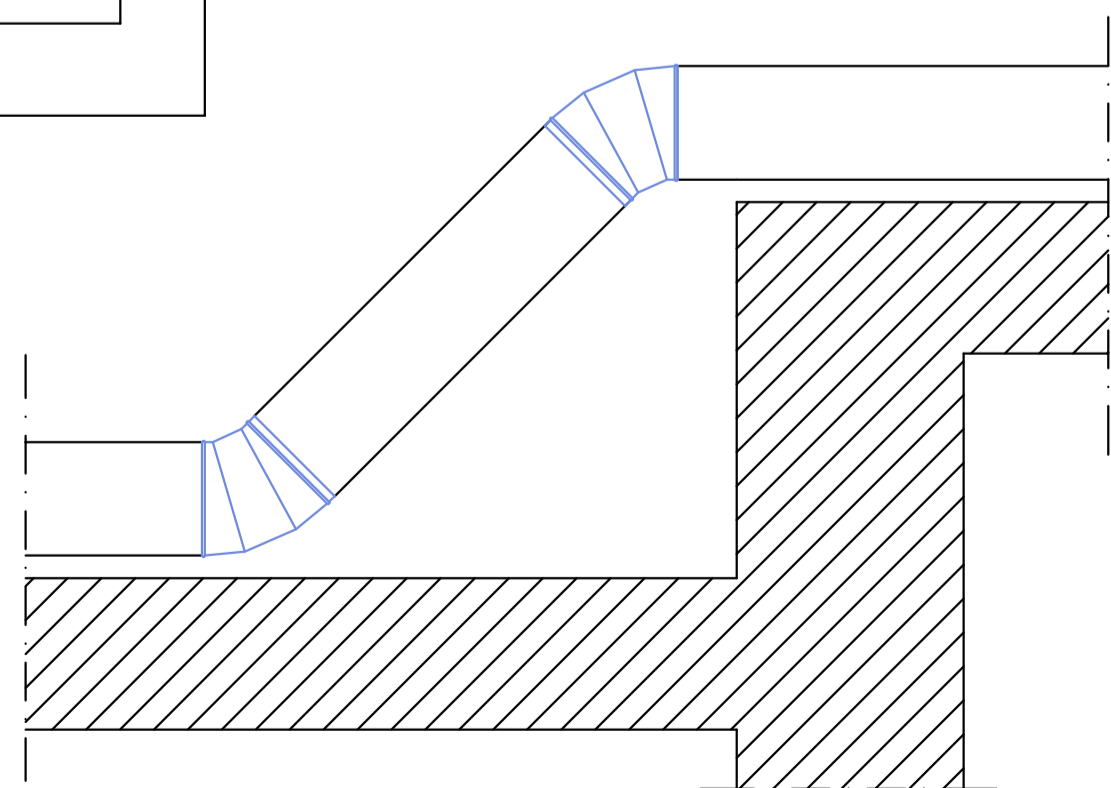
PARTICOLARE SUPERAMENTO DEL DISLIVELLO TRA SOLAI Scala 1:10
