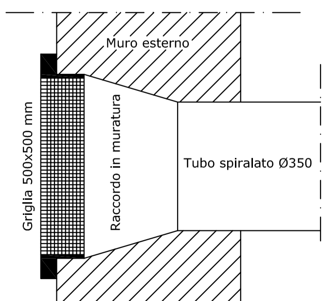
PARTICOLARE DI PRESA ED ESPULSIONE ARIA A PARETE Scala 1:10
