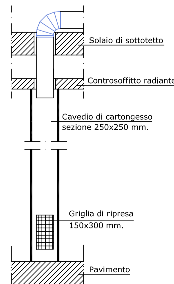
PARTICOLARE "A" Scala 1:20
