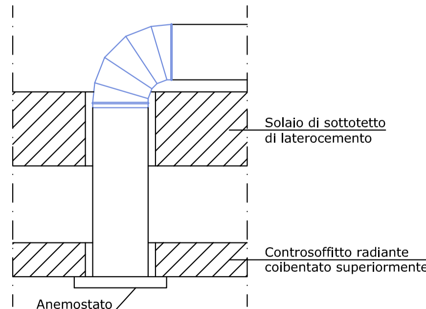
PARTICOLARE COLLEGAMENTO DEGLI ANEMOSTATI Scala 1:10
