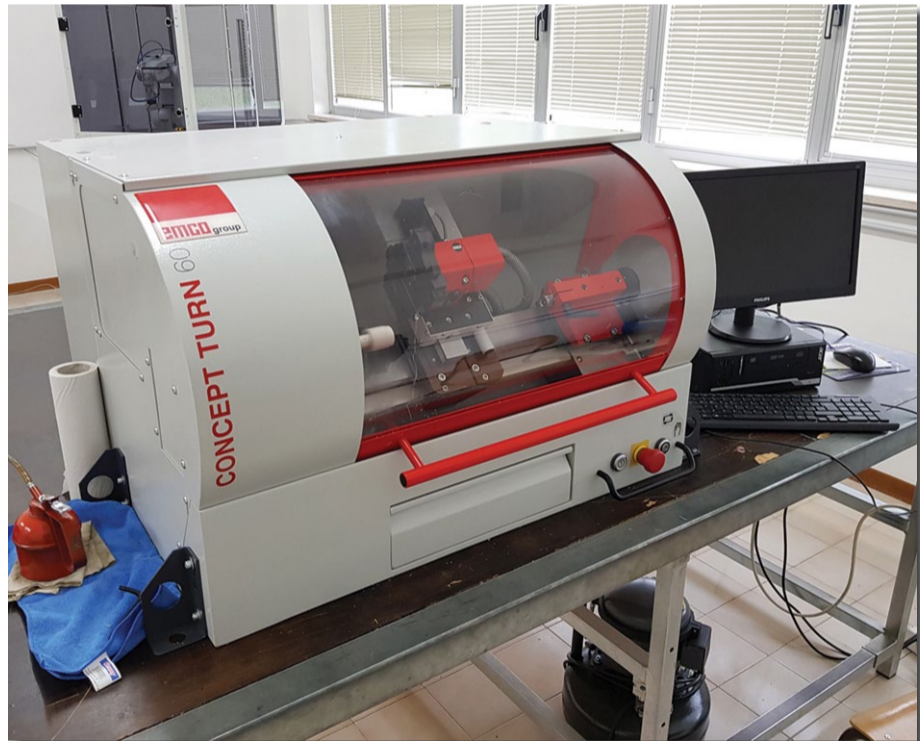
Qui sopra un tornio a controllo numerico. Sotto un robot antropomorfo
